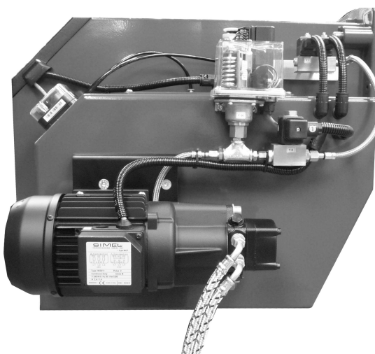
Насосная станция для МК2.1 / МК2.2
